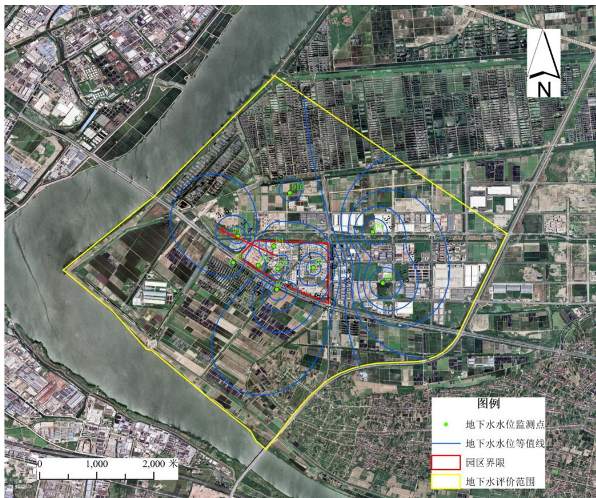
图 6.3.1-3 地下水等水位线图
