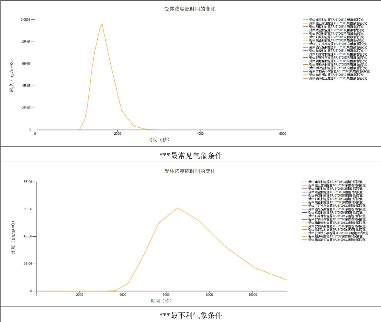
图 6.6.6-6 关心点有毒有害物质浓度随时间变化情况
