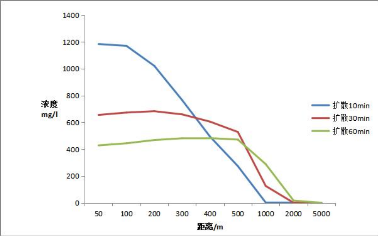
图 6.6.6-7 不同扩散时间条件不同距离处浓度值
