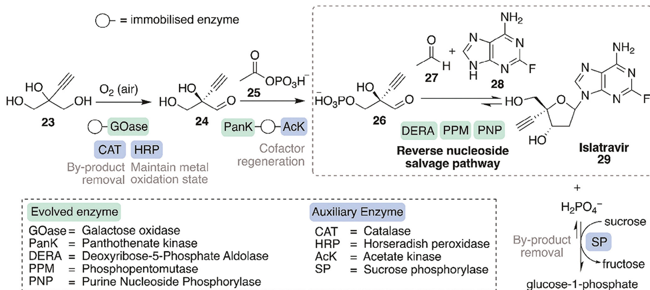
方案8.生物催化级联用于生产药物islatravir
