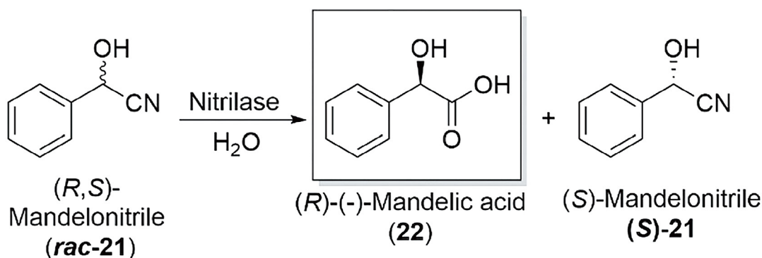
方案7.腈水解酶工业化生产重要的药物前体(R)-扁桃酸(22)
